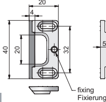
Striker plate
