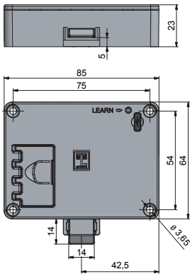
RFID-Leser L033-A01
