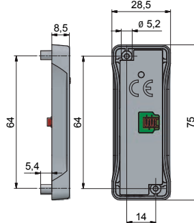
RFID-Leser L033-A02
