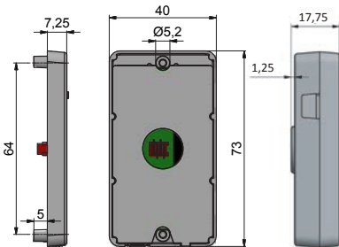
RFID-Leser L033-A01
